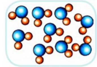
Su
