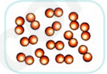
Hidrojen
