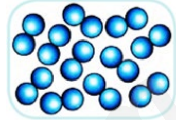
Oksijen
